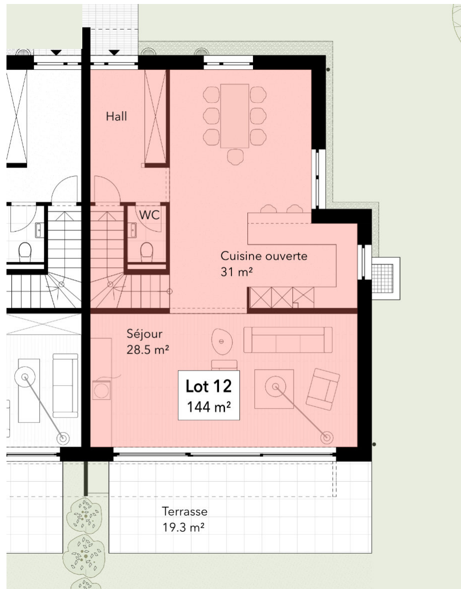
Rez-de-Chaussée
